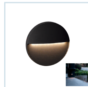
HLO-5564 (3W) Size : Ø160x31mm
